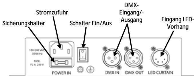
Bedienfeld Oberseite
